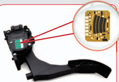
2. Pedal de aceleración con potenciómetro incorporado (sin cable).
